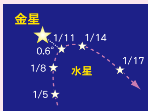
【金星に対する水星の動き】
