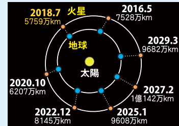
【地球と火星の最接近時の位置関係】
